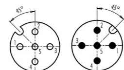
Mastkabel für Gabelstapler M12A-5p (Stecker/Busche) Mast cable for Forklift M12A-5p (Male/Female)
